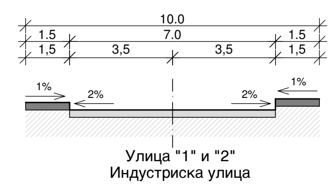
ПРЕСЕК А - А
